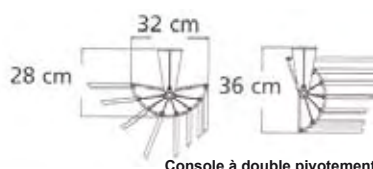
Console à double pivotement
