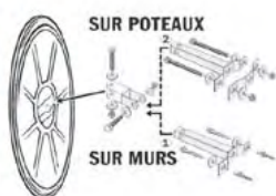
Fixation pour murs et poteaux de 34 à 90 mm de section
